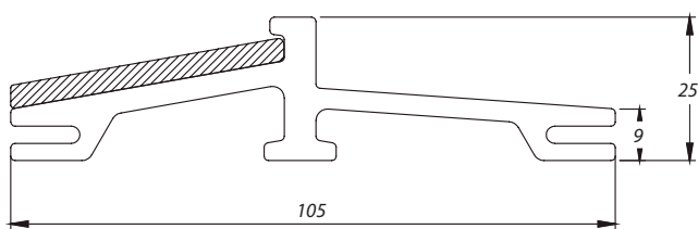
TVÄRSNITT 25 MM TILLGÄNGLIGHETSANPASSAD TRÖSKEL DURABEL MED EKBELAGD INSIDA
