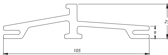
TVÄRSNITT 25 MM TILLGÄNGLIGHETSANPASSAD TRÖSKEL DURABEL
