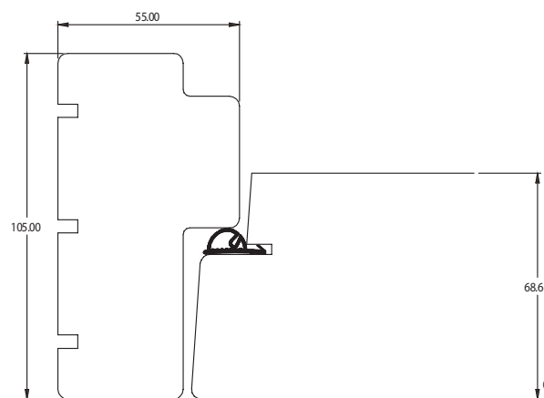
KONSTRUKTION BRANDHÄMMANDE 45 MIN
