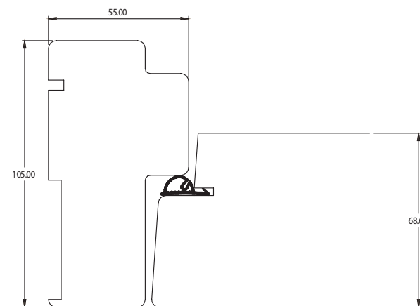
KONSTRUKTION SÄKERHETSKLASS RC3
