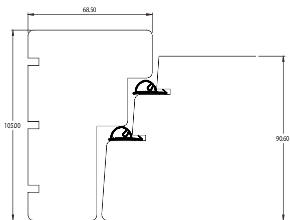
KONSTRUKTION PASSIV 91
