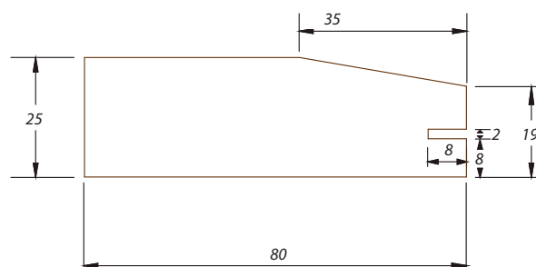
TVÄRSNITT TRÖSKEL EK PIVOTHÄNGD YTTERDÖRR
