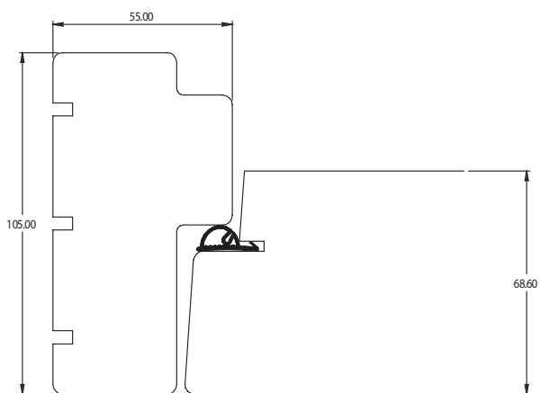
KONSTRUKTION BRANDHÄMMANDE 30 MIN
