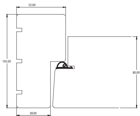
PIVOTHÄNGD YTTERDÖRR
