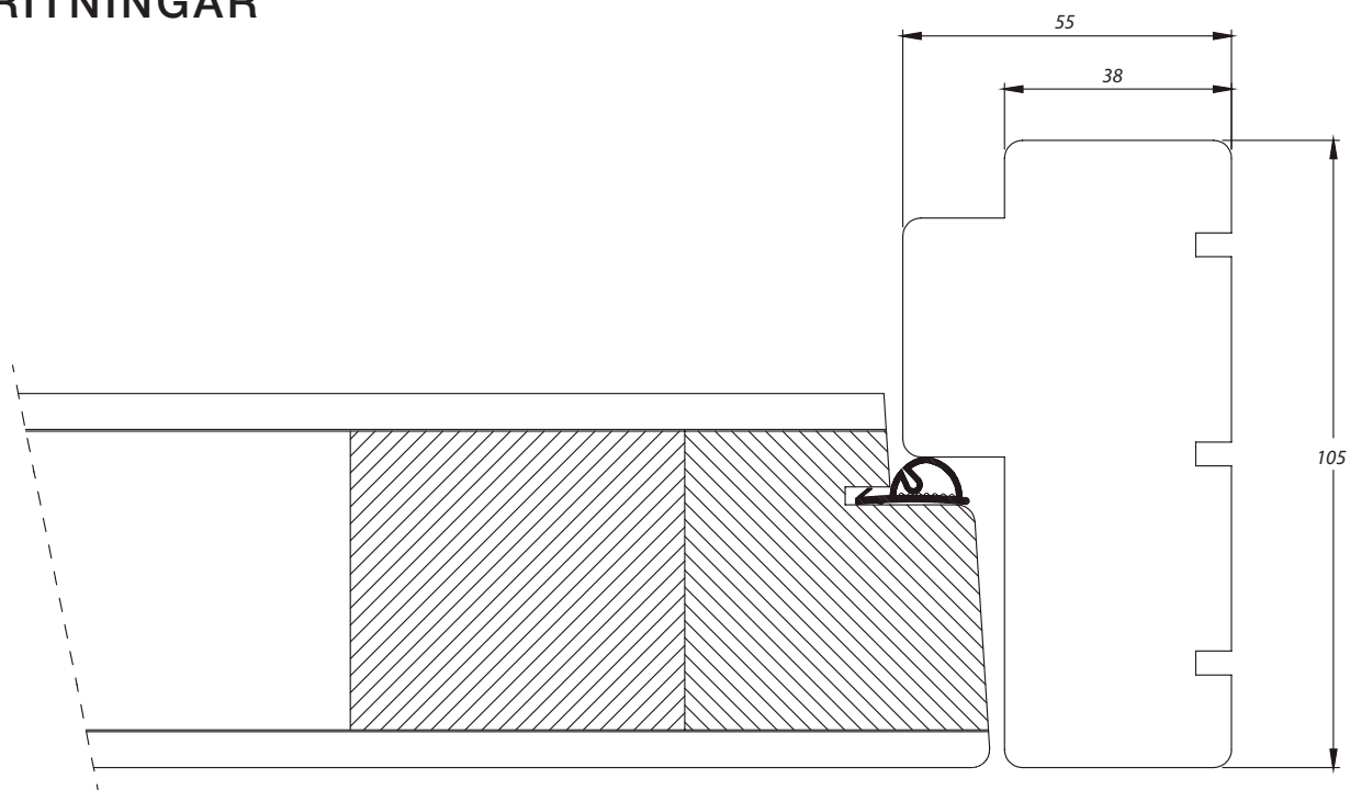
TVÄRSNITT MÅLAD SLÄT YTTERDÖRR MED KARM
