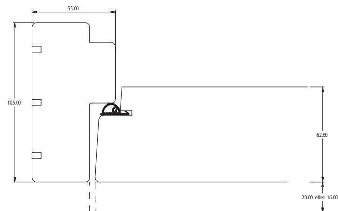
FASADBELÄGGNING INTEGRERAD PÅ DÖRR OCH KARM
