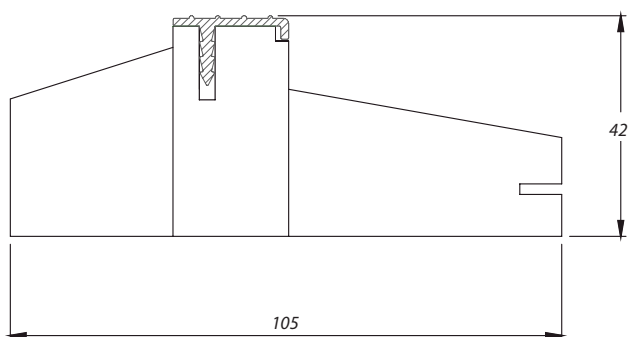
TVÄRSNITT YD TRÖSKEL EK UTÅTGÅENDE
