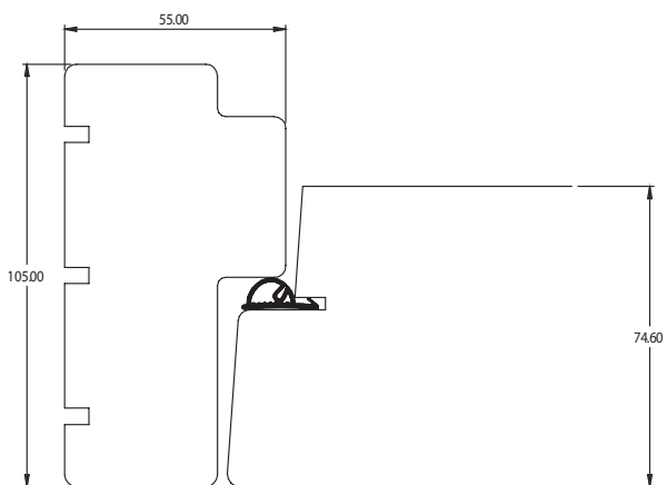
KONSTRUKTION BRANDHÄMMANDE 60 MIN
