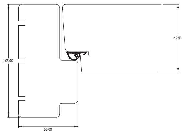
INÅTGÅENDE YTTERDÖRR
